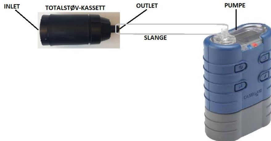
Figur 1: Oppsett av totalstøv-filterkassett for måling av totalstøv. Pumpen kobles til filterkassetten ved hjelp av en slange. Slangen går mellom pumpen og outlet -åpningen på filterkassetten.
